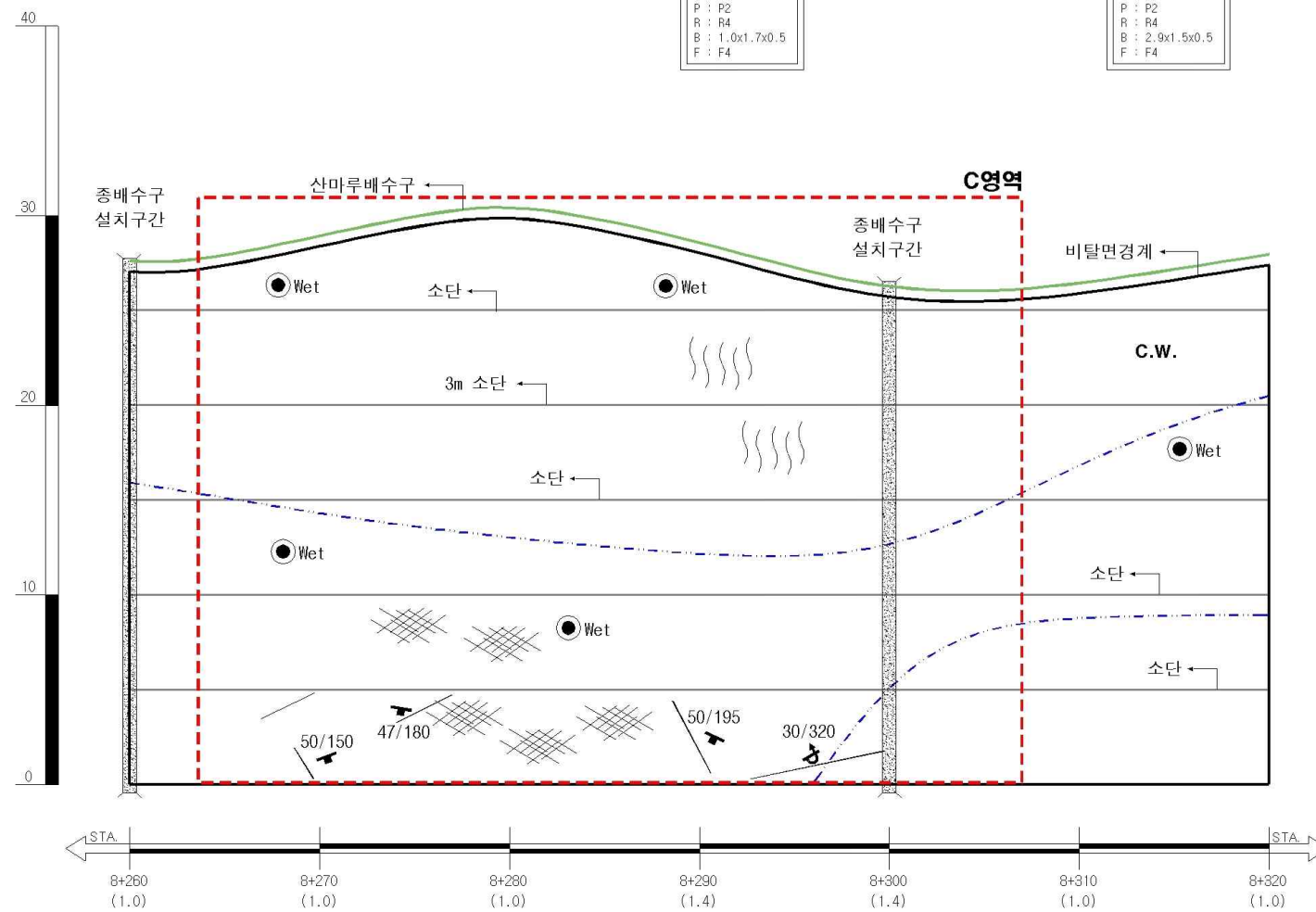
<A-A' 단면>
