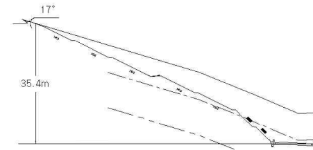
<A-A'단면>
