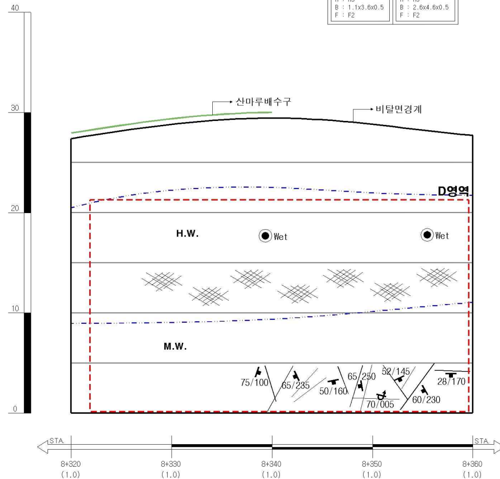
<A-A'단면>
